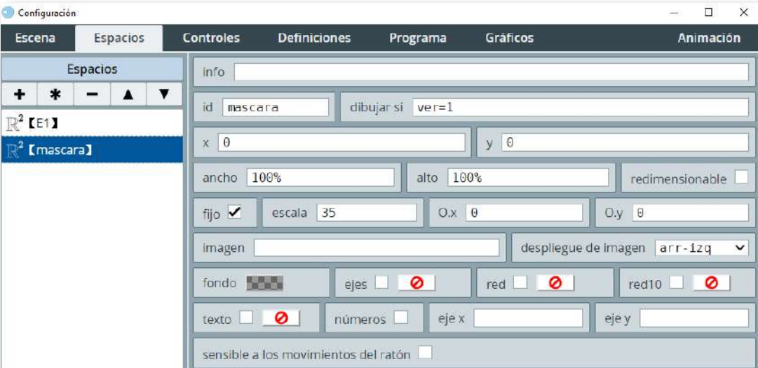
Figura 1.5. Espacio transparente que evita hacer clic sobre las respuestas
