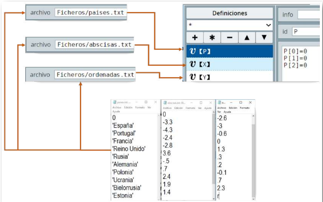
Figura 1.8. Asignación de datos externos a los vectores P , X e Y .
