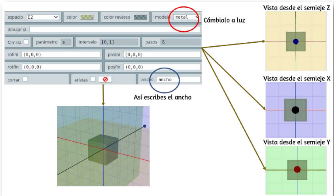
Figura 2.2. Gráfico cubo agregado al espacio 3D con los planos cartesianos XY , YZ y ZX .
