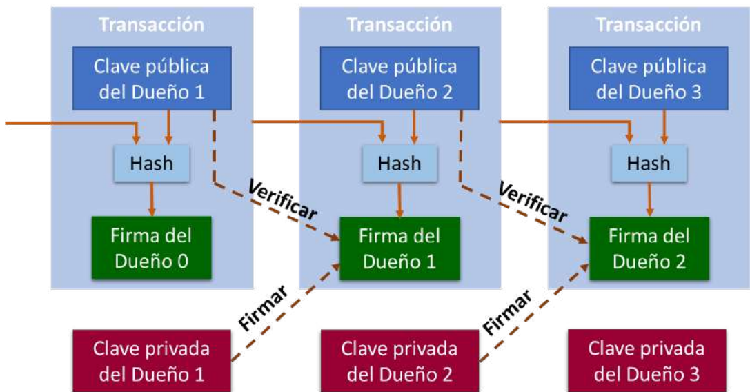
Figura 6.1. Transacciones, según el white paper de Nakamoto. Cada dueño transfiere la moneda al próximo al firmar digitalmente un hash de la transacción previa y la clave publica del próximo dueño y agregando estos al final de la moneda. Un beneficiario puede verificar las firmas para verificar la cadena de propiedad.
