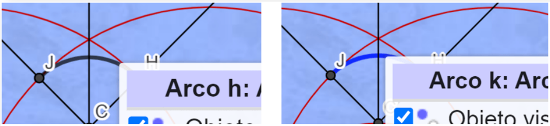
Figura 6.3. Arcos de circunferencia de la primera tarea.
