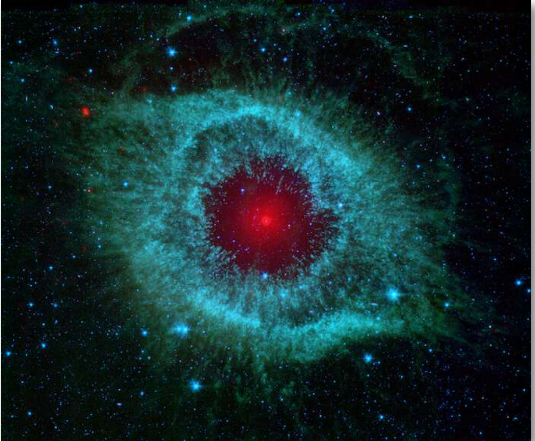
Figura 2.4. Esta imagen puede parecer un globo ocular espeluznante, ¡pero en realidad es una nebulosa! El Telescopio Espacial Spitzer de la NASA capturó esta imagen de la Nebulosa Helix, que se encuentra en la constelación de Acuario. Crédito de imagen: NASA/JPL-Caltech/Universidad de Arizona.
